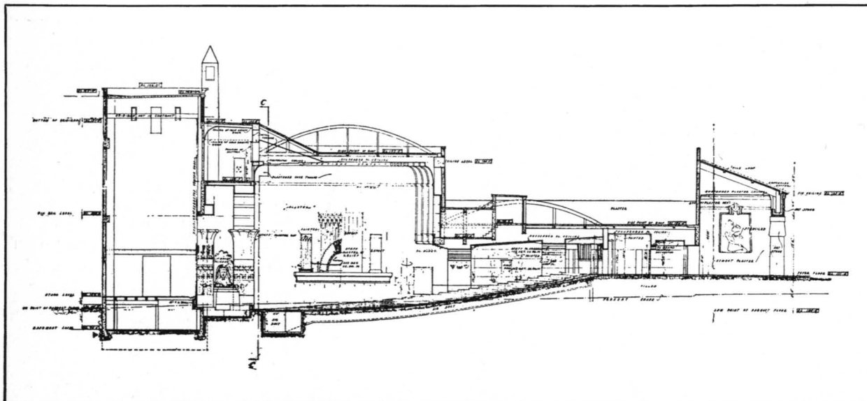
LONGITUDINAL SECTION
