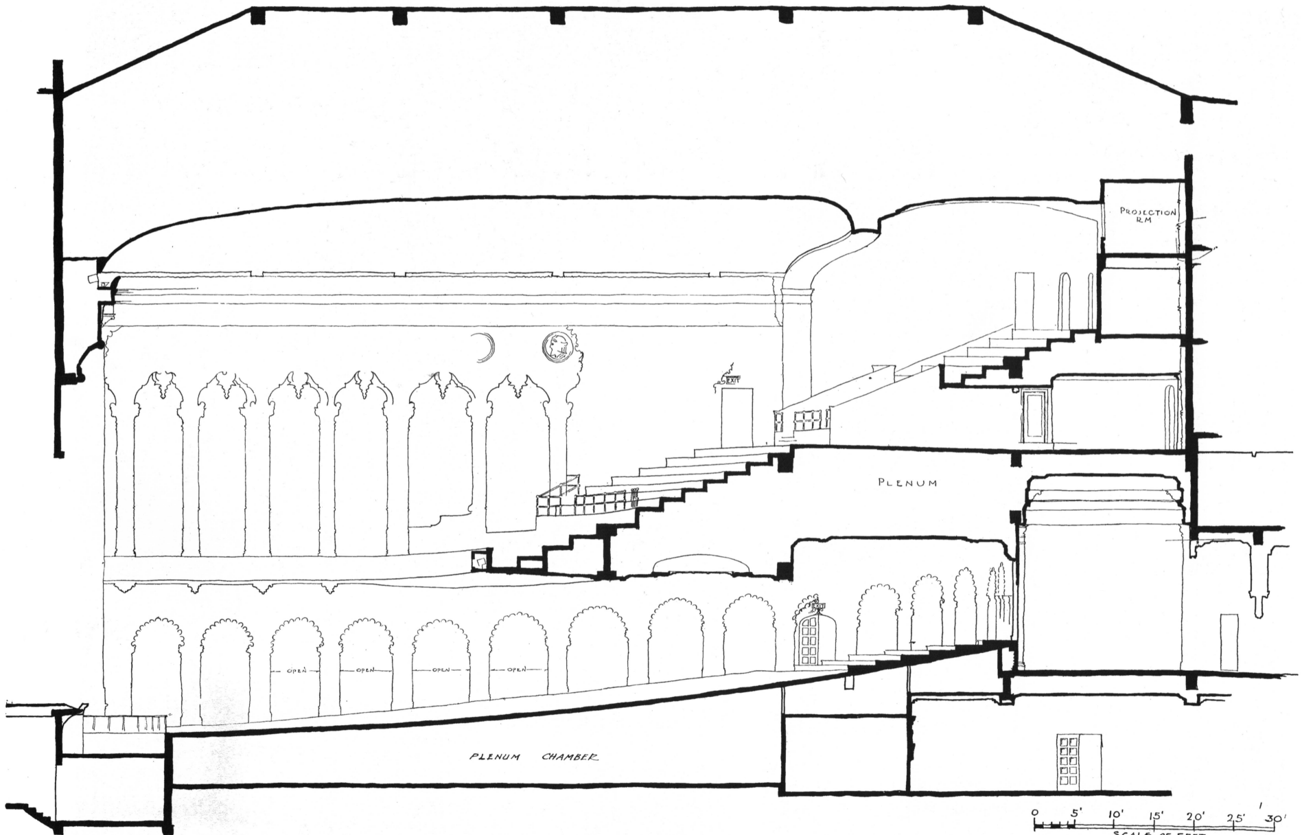
LONGITUDINAL SECTION
